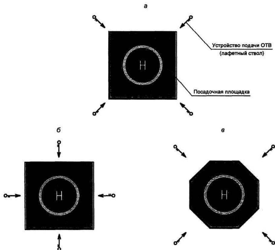
а - диагональное размещение; б - линейное; в - радиальное Рисунок А.1 - Схемы размещения стационарных лафетных стволов
